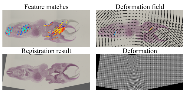
図 4: スパースカーネル回帰による変形場のモデル化に基づいた画像位置合わせ.
