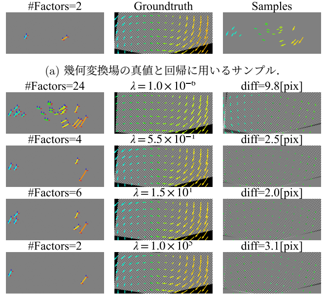
(a) 幾何変換場の真値と回帰に用いるサンプル。 (b) さまざまな \lambda に対して推定された因子とそこから生成された幾何変換場、および真値との差分。
