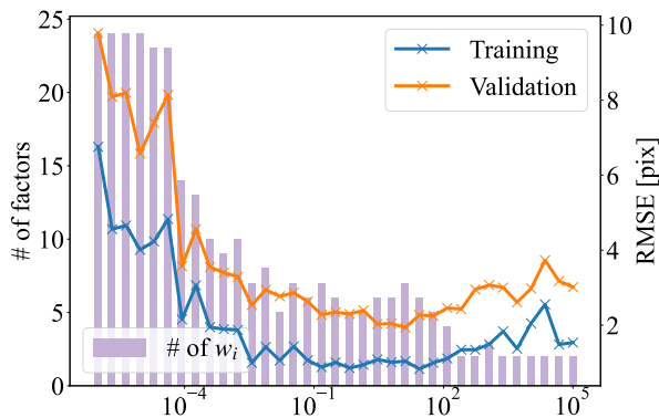
図 3: さまざまな \lambda に対する RMSE と因子数の変化.
