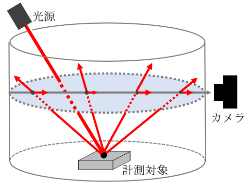
図 5 観測値は観測方向に向かう散乱光強度の積算値
