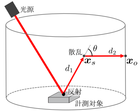
図 4 単一散乱による反射光の散乱光の観測モデル
