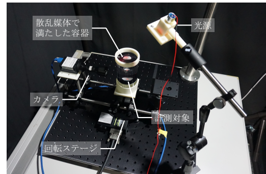
図3 観測システム
