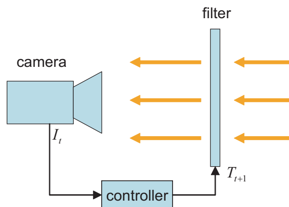
図1 システムのモデル
