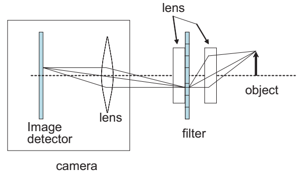
図3 改良システムのモデル図
