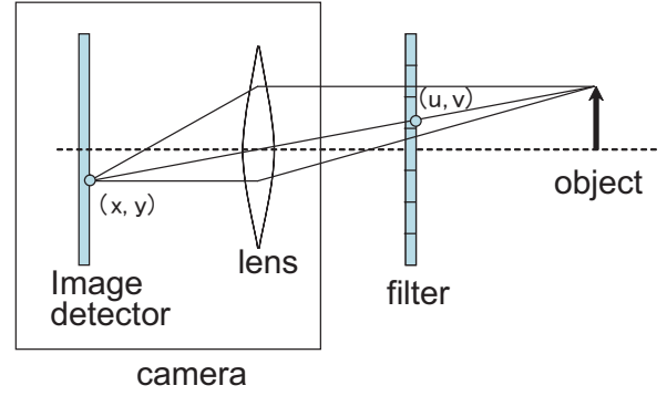
図2 システムの幾何モデル
