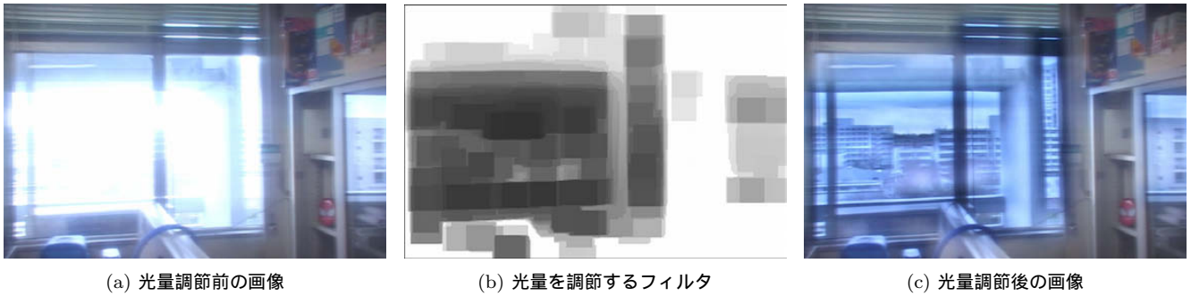
図 16 システムを用いた屋内からの窓の外の撮影
