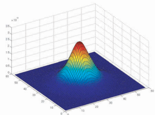
図 13 ぼけ関数
